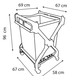
Estructura plegable que permite ahorrar espacio.
